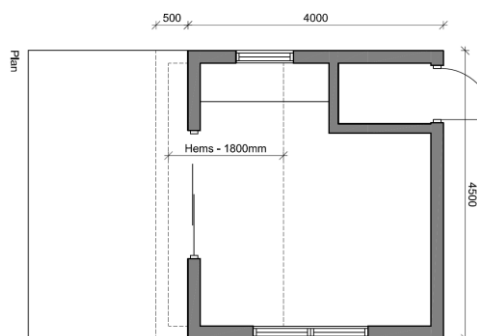
Grundplan – stilplet del (hemsudhæng) må ikke opføres
