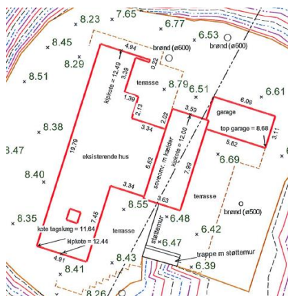
Eksisterende forhold
