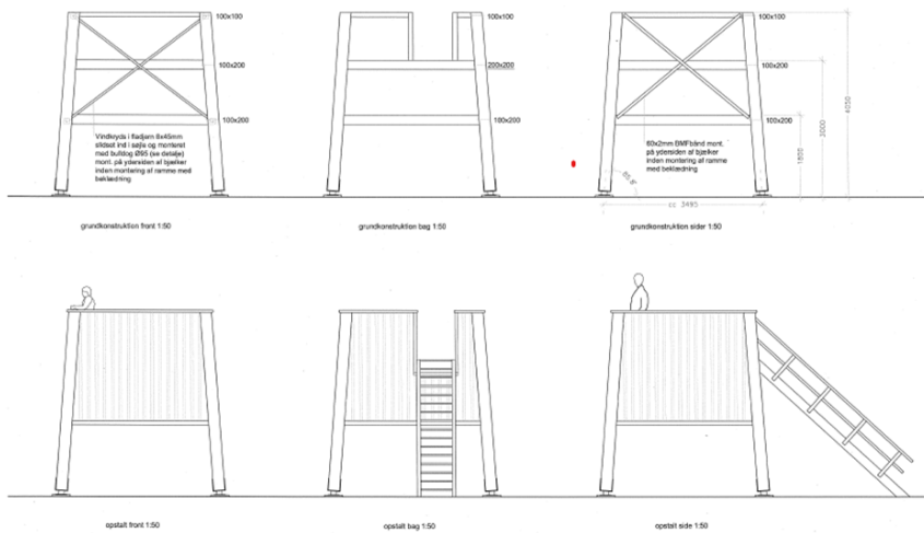
Figur 2, tegning af tårnet, fra ansøgningen
