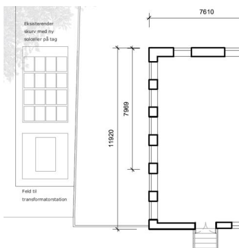
Eksisterende forhold med byggefelt samt placering af solceller og transformator (vist under)
