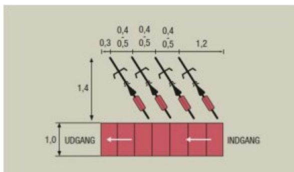
Skematisk aftegning af Aarhus Kommunes retningslinjer for cykelstativer.
