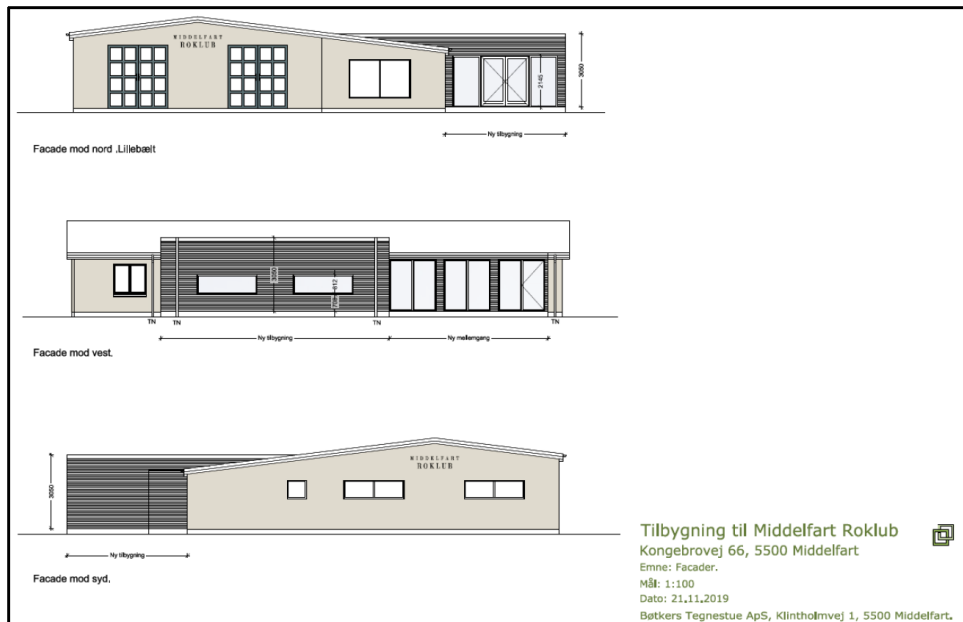
Fig. 3. Tilsendt fra ansøger. Tegning af bygningens facader efter ombygningen.
