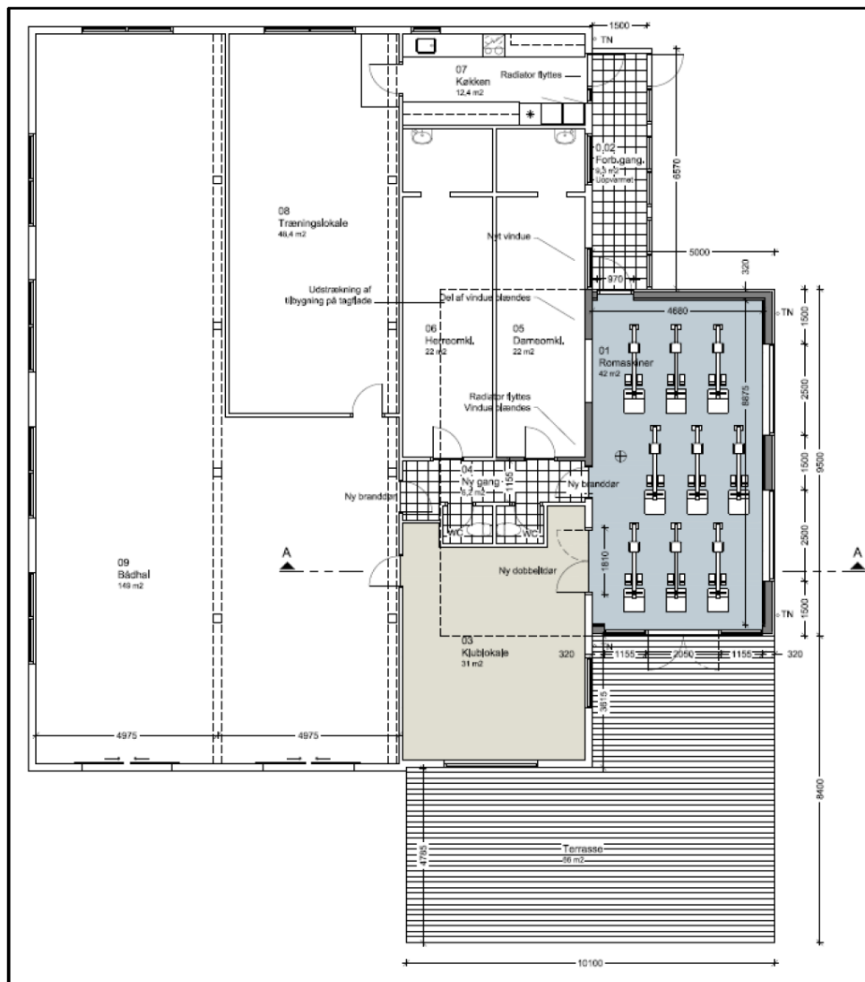
Fig. 4. Tilsendt fra ansøger. Forbindelsesgangen ses øverst til højre og ergometerrummet under dette. Terrassen er i tegningens nederste højre hjørne.
