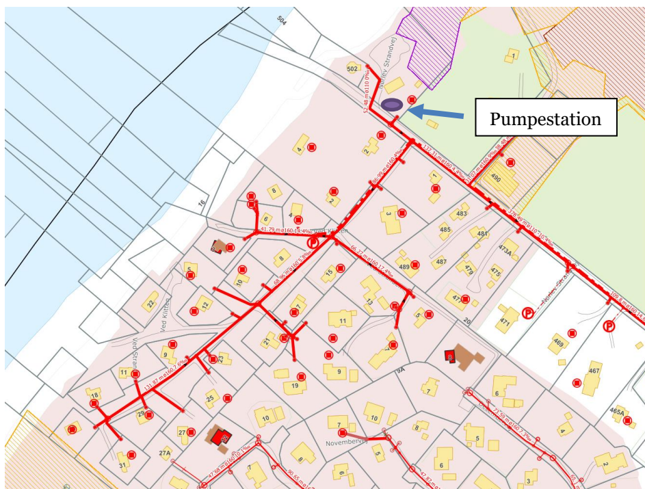
Fig. 3 er en medsendt situationsplan over projektet med en markering af, hvor de nedgravede kloakledninger, brønde og pumpestationen placeres.
