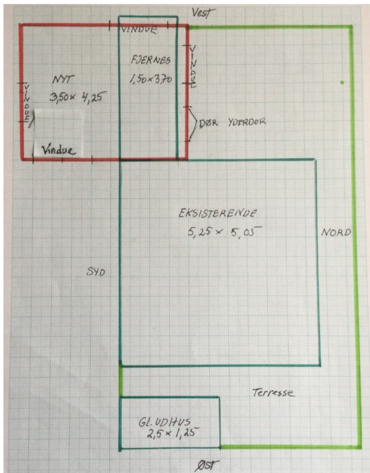
Figur 3, plantegning fra ansøgning. Med rødt nyopføres som tilbygning. Det grønne, markeret "Fjernes" nedrives.
