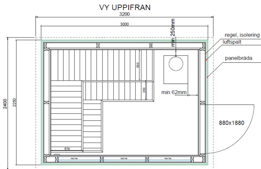
Figur 5, plantegning fra ansøgning
