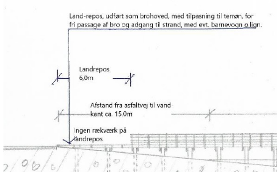
Fig. 2. Længdesnit fra ansøgningen, der viser asfaltervej, landrepos og begyndelsen af badebroen.
