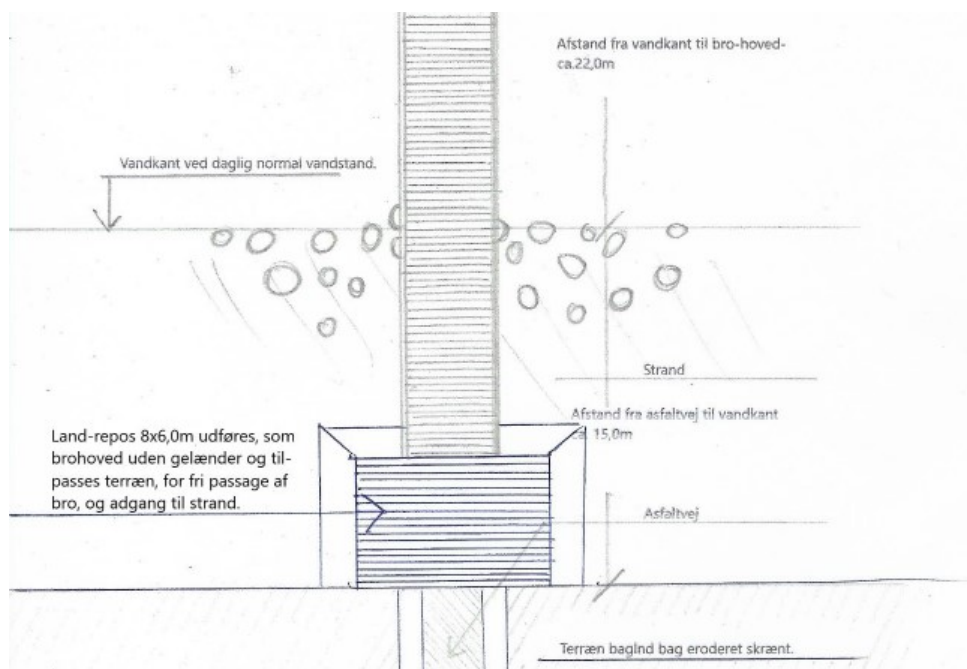
Fig. 3. Principtegning fra ansøgningen, der viser landrepos (nederst) samt begyndelsen af badebroen
