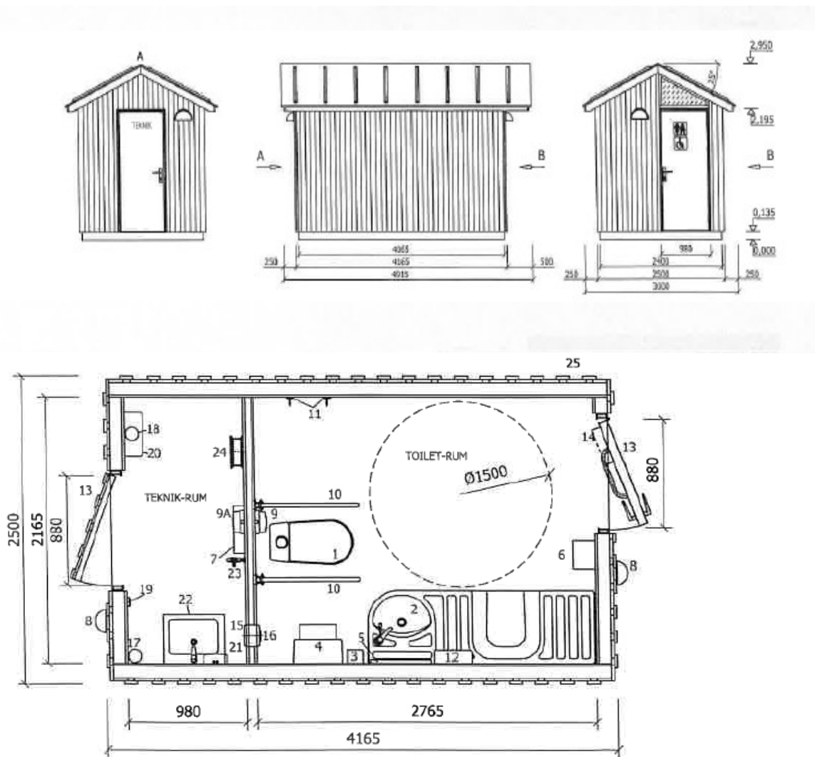
Fig. 5. Fremsendte tegninger og mål vedrørende ny toiletbygning.
