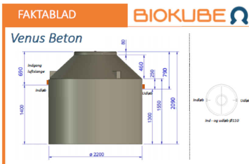
Fig. 3. Fremsendte tekniske detaljer for minirenselanlægget.
