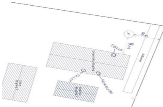
Fig. 2. Fremsendt tegning, der viser placeringen af minirenselanlægget.
