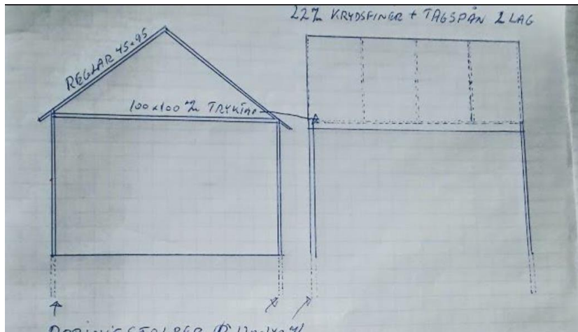
Figur 3. Skitsetegning af den ansøgte bålhytte. Materiale fra ansøgningen.
