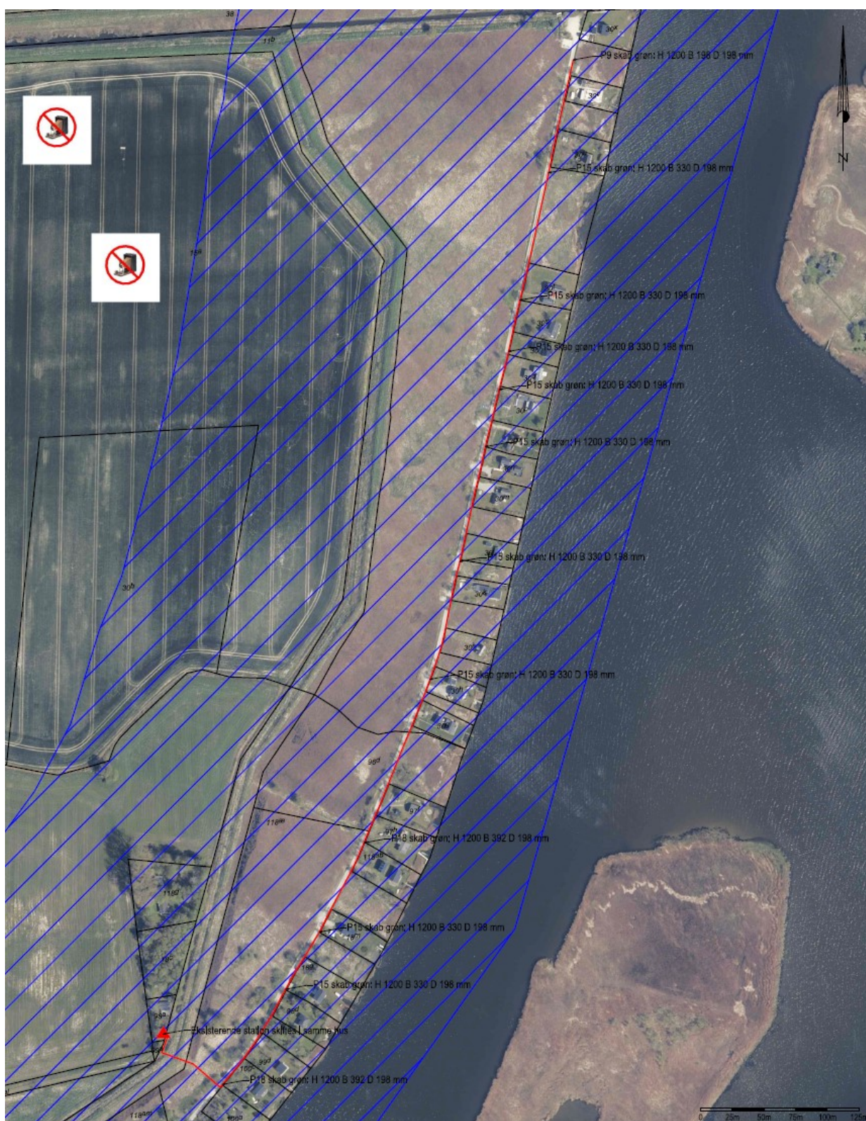
Plan viser kabeltracéet. Mod syd kobles til en eksisterende transformerstation (rød trekant). Teknikskabe er markeret med sorte pile og står langs vejen.
