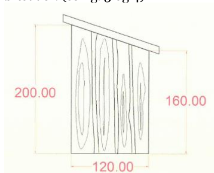
Fig. 3 medsendt tegning af muldtoilet
