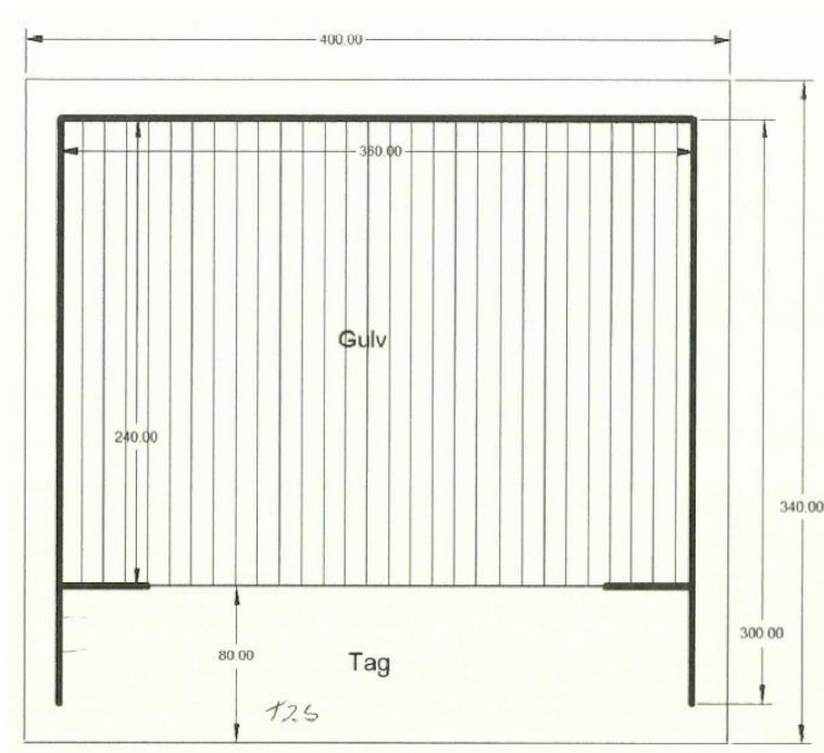
Fig. 5 og 6 medsendt tegning med mål på shelteret.
