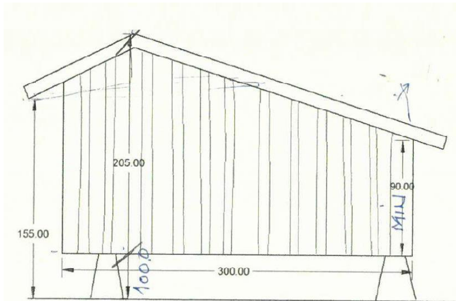
Fig. 5 og 6 medsendt tegning med mål på shelteret.
